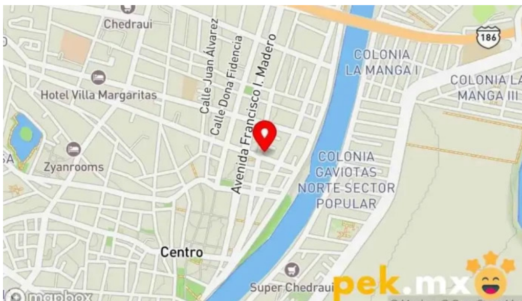
Hct mapa
